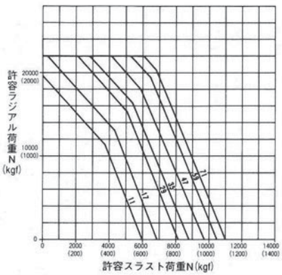
[NE枠] 許容ラジアル・スラスト荷重
