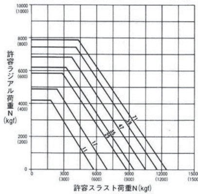
[C枠] 許容ラジアル・スラスト荷重
