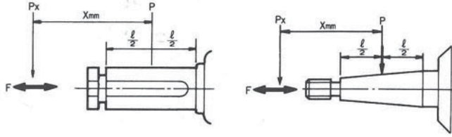
[B枠] 許容ラジアル・スラスト荷重
