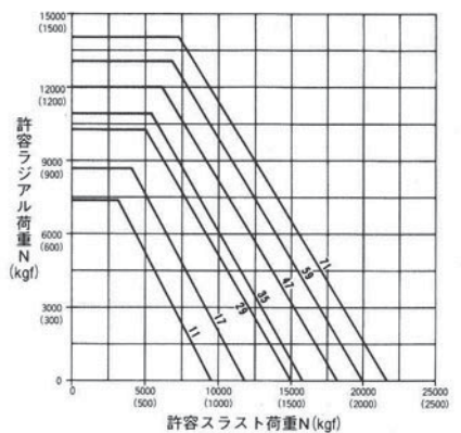
[D枠] 許容ラジアル・スラスト荷重
