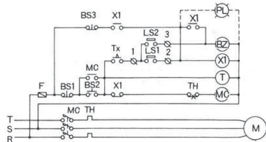
[モートル電源遮断及び警報回路例]
