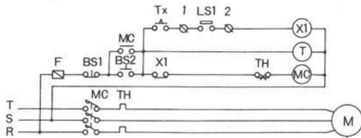
[モートル電源遮断回路例]
